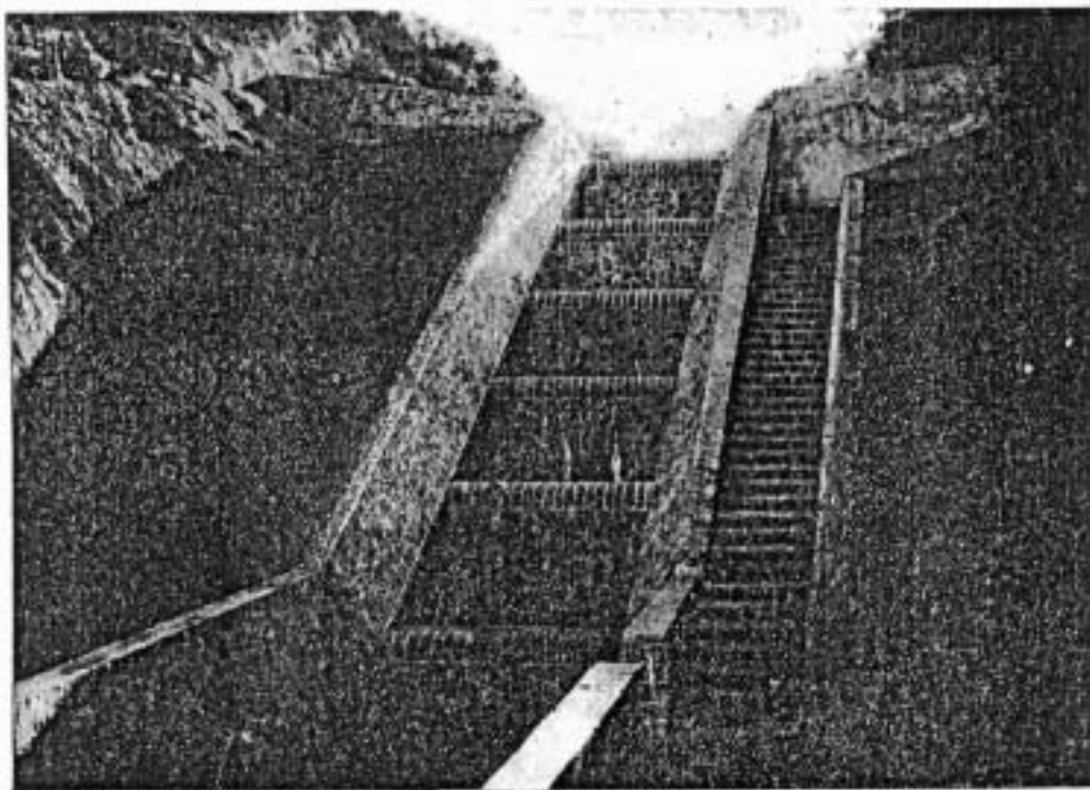
Fig. 11. — Briglia a snlti successivi.
